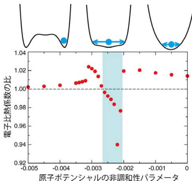
図 2：原子の質量を 5% 増やしたときの電子比熱係数の比の計算結果。原子ポテンシャルの形を変えて計算しているが、ポテンシャルの底が平らで原子の振幅が大きくなる水色の領域で電子比熱係数は減少する。
