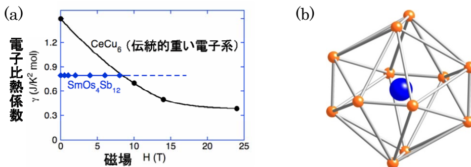
図 1 : (a) \text{CeCu}_6 と \text{SmOs}_4\text{Sb}_{12} の電子比熱係数を磁場の関数として描いたもの。自由電子系の電子比熱係数は \text{mJ/K}^2\text{mol} のオーダーである。(b) 12 個の Sb 原子(オレンジ)の 20 面体のカゴに内包される Sm 原子(青)。Sm 原子がカゴの中のスペースで振幅の大きな振動をする。
